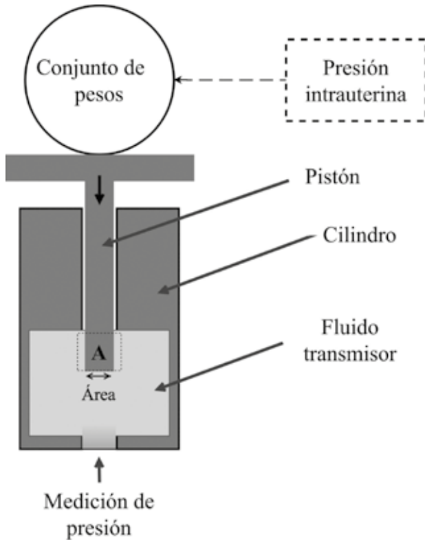
Figura 3. Calibración de presión por medición indirecta
