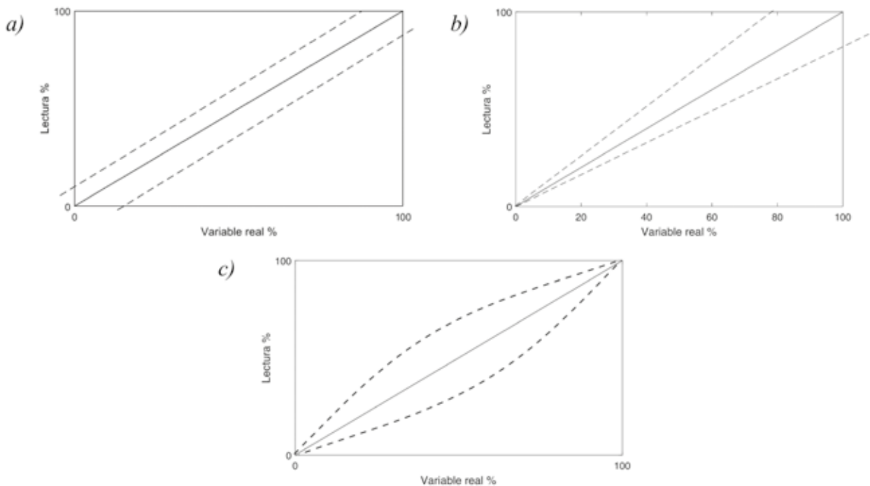
Figura 2. a) Error de cero, b) Error de multiplicación, c) Error de angularidad
