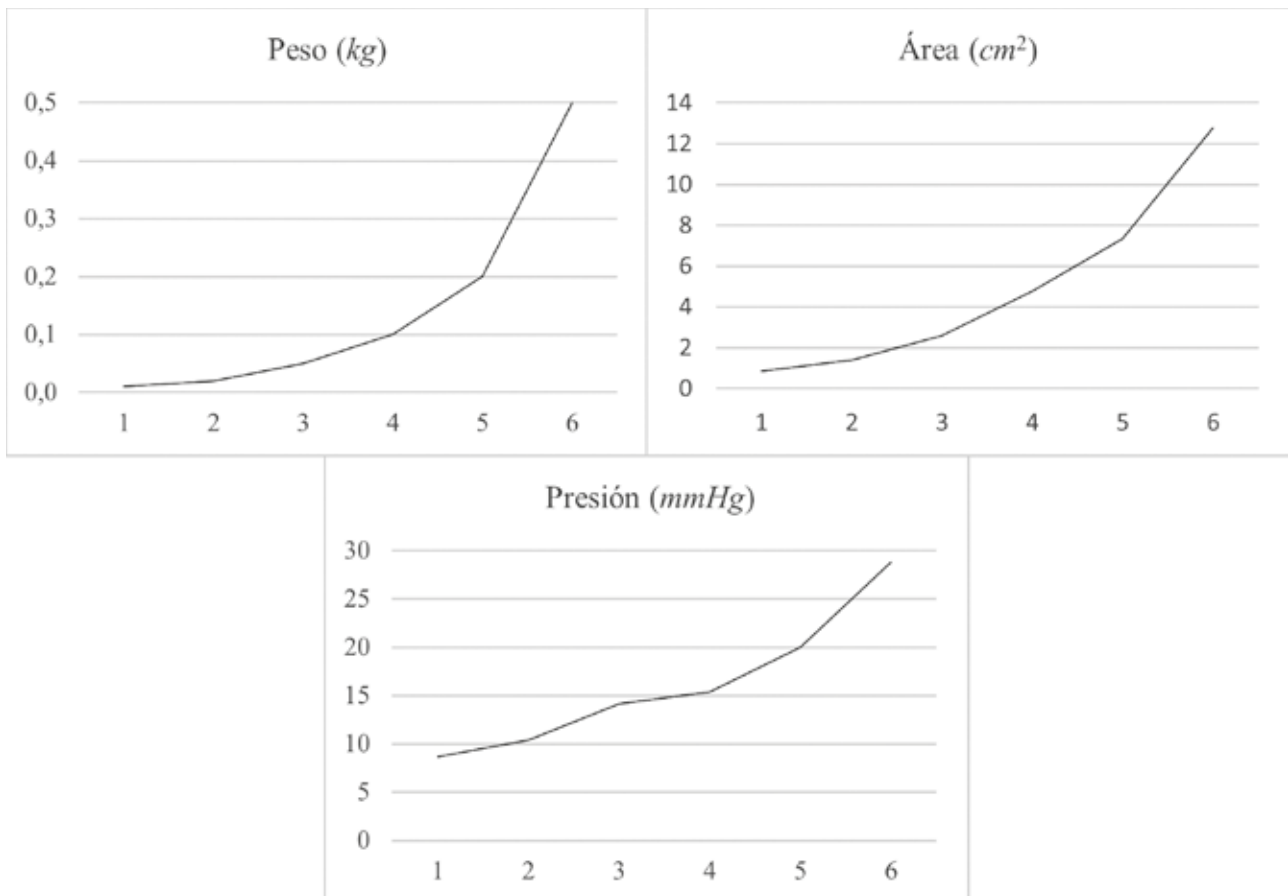
Figura 4. Resultados de medición para procedimiento de calibración por peso muerto
